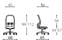
Base 5 razze senza braccioli
