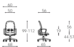
Base 5 razze c/braccioli fissi N10
