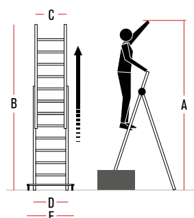
Gradino 30x30 mm. Rung 30x30 mm.
